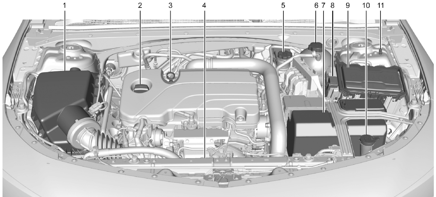
Рядный 4-цилиндровый двигатель с турбонаддувом объемом 1,5 л
